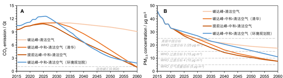
图 2.3 大气环境质量降碳减污协同治理中长期路线示意（A：CO 2 排放，B：PM 2.5 浓度）
