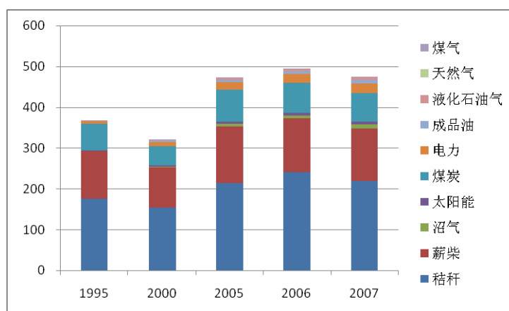
图 3.4 1995~2007 年全国农村人均生活用能分品种变化趋势
