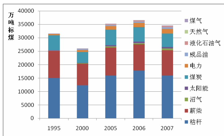
图 3.3 1995~2007 年中国农村生活用能分品种及总量的变化趋势
