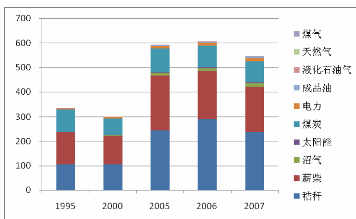
图 3.6 1995~2007 年西部地区农村人均生活用能分品种变化趋势
