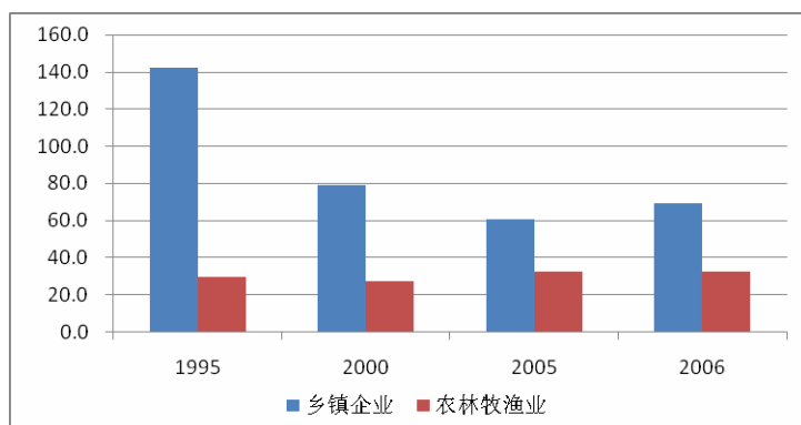
图 3.9 1995~2007 年农林牧渔业和乡镇企业单位增加值终端能源消费强度
