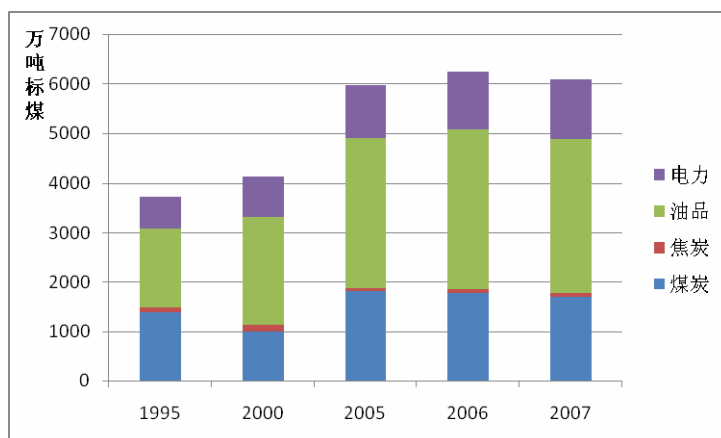
图 3.8 1995~2007 年中国农林牧渔业终端用能分品种及总量的变化趋势
