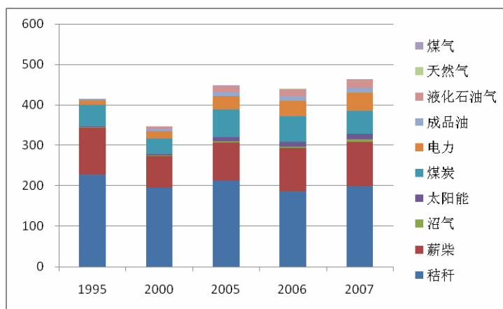
图 3.5 1995~2007 年东部地区农村人均生活用能分品种变化趋势
