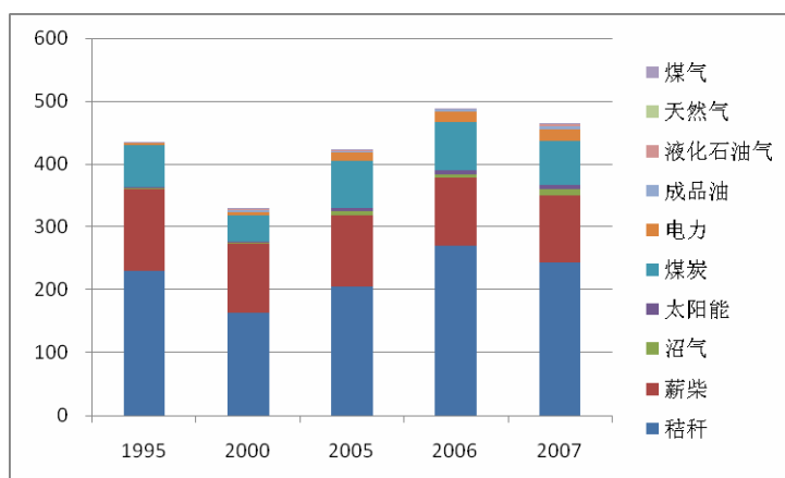
图 3.7 1995-2007 年中部地区农村人均生活用能分品种变化趋势
