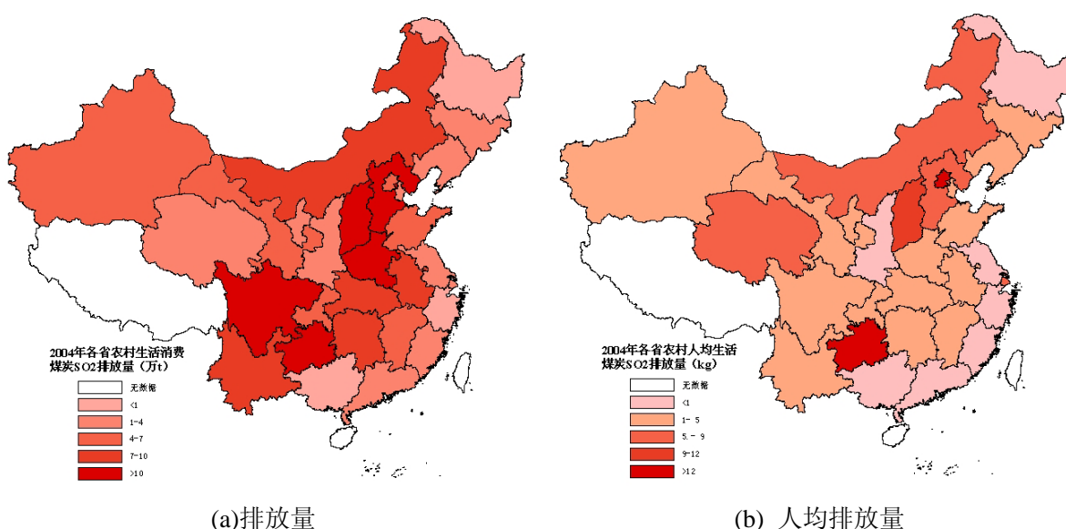
图 4.1 2004 年各省农村生活消费煤炭 SO 2 排放总量与人均排放量
