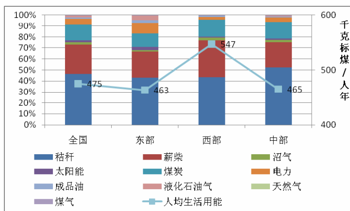
图 3.1 2007 年分地区农村人均生活用能及品种构成
