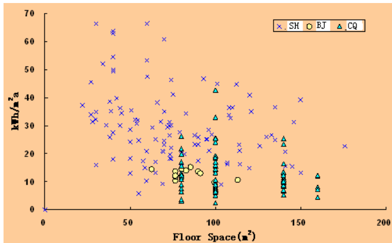
图 2-12 住宅能耗比较（北京、上海、重庆）
