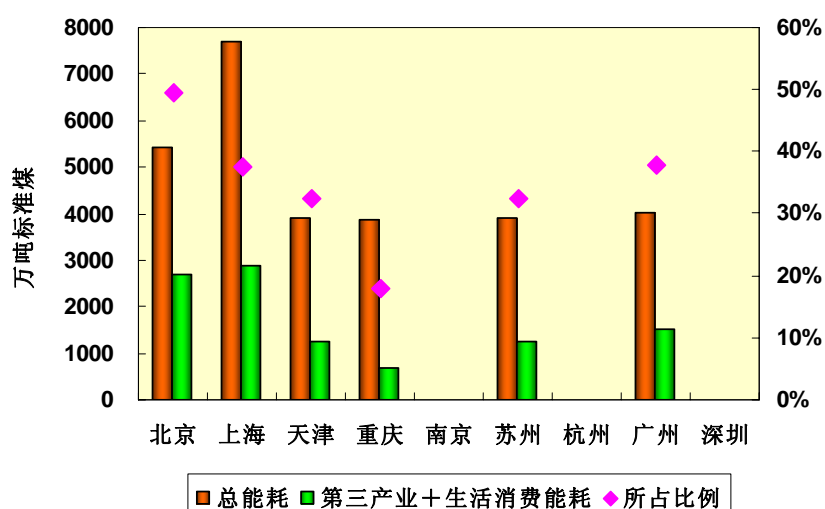
图 2-3 各地第三产业及生活消费能耗（2005）
