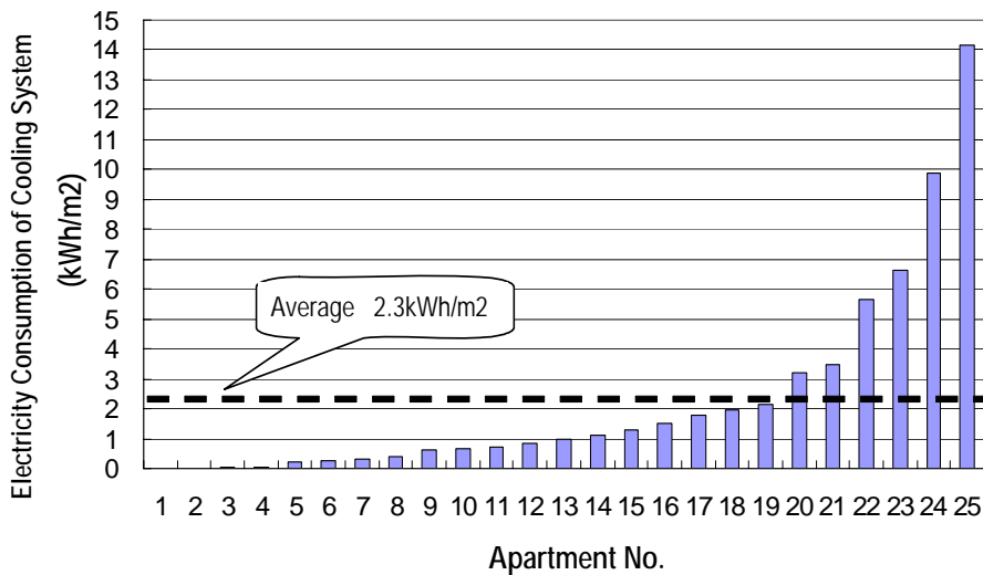
图 2-13 北京某采用分体空调的住宅楼各住户全年空调能耗 (kWh/m 2 .年)
