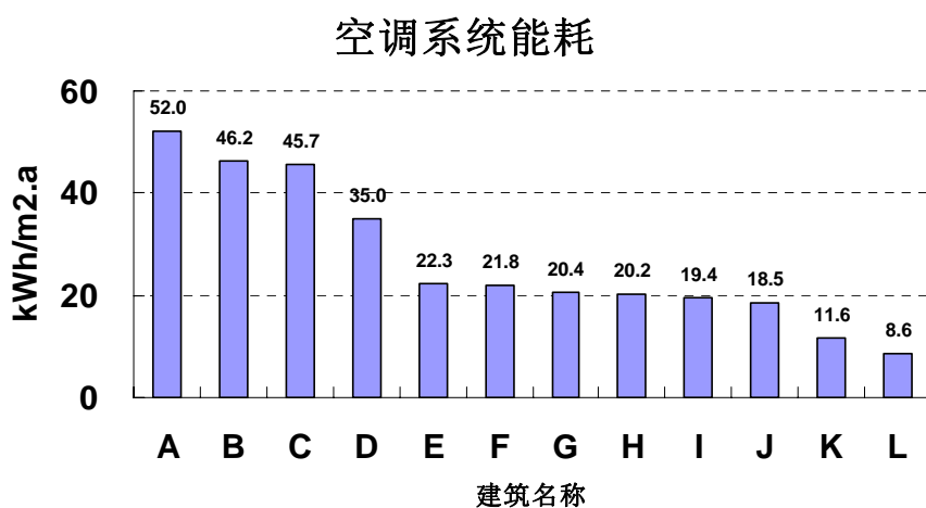
图 2-11 位于北京的一些政府机构办公大楼的空调电耗 (单位: kWh/m²·年)
